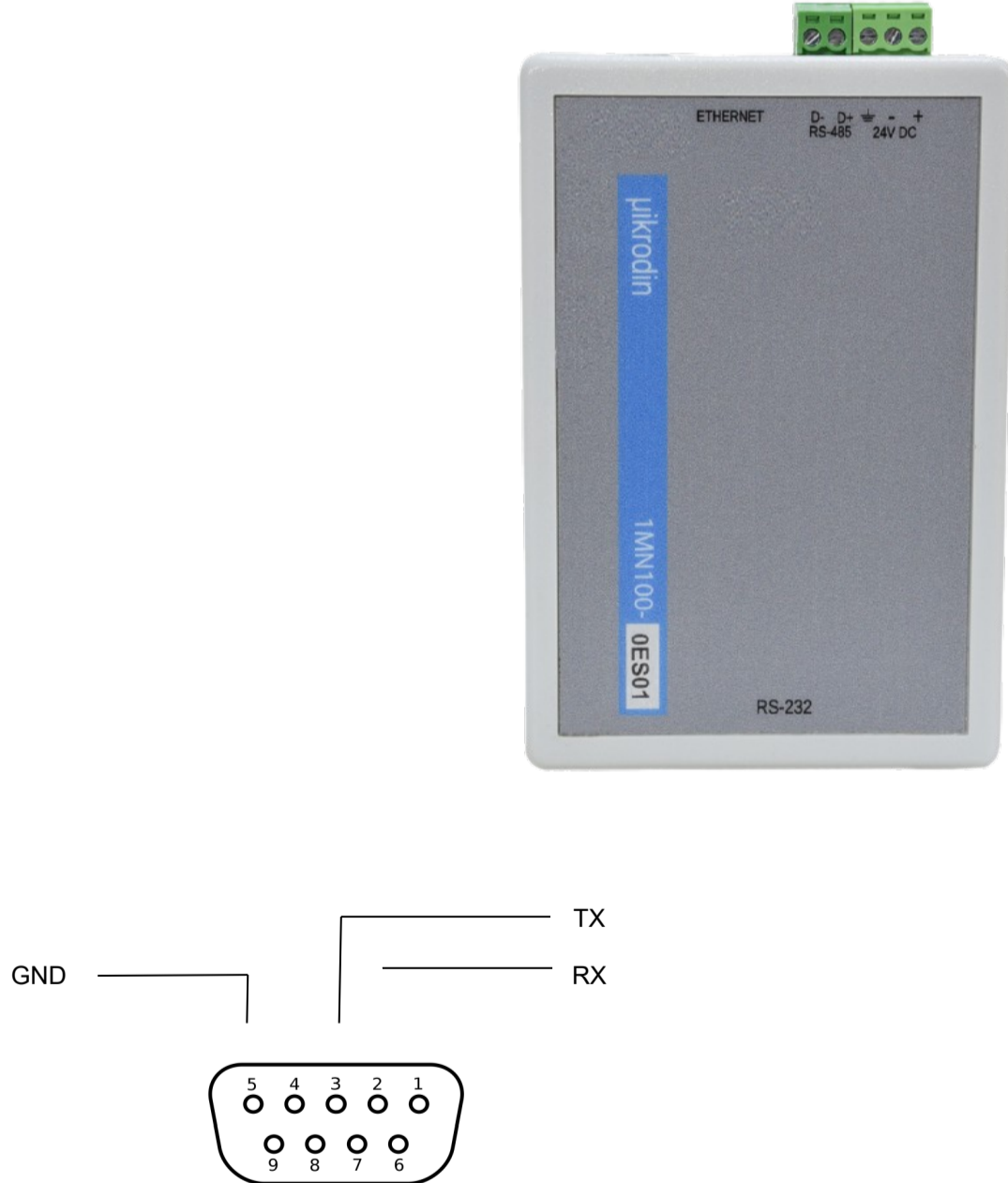
1MN 100-0ES01 Dönüştürücü Görünümü
